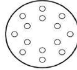
GLS 6 Ø 150 mm 8 db Ø 10 mm elszívólyuk Ø 118 mm lyukkörön 6 db R 10 mm elszívólyuk Ø 80 mm lyukkörön
