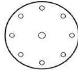
GLS 1 Ø 150 mm 8 db Ø 10 mm elszívólyuk Ø 120 mm lyukkörön + 1 db 17 mm központi lyuk
