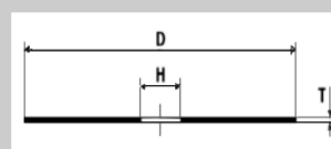
Forma BF41: egyenes
