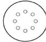
GLS 2 Ø 150 mm 8 db Ø 10 mm elszívólyuk Ø 65 mm lyukkörön
