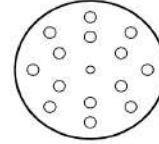
GLS 6 Ø 150 mm 8 db Ø 10 mm elszívólyuk Ø 118 mm lyukkörön 6 db Ø 10 mm elszívólyuk Ø 80 mm lyukkörön + 1 db 7 mm központi lyuk
