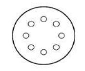
GLS 4 Ø 115 mm 8 db Ø 10 mm elszívólyuk Ø 65 mm lyukkörön
