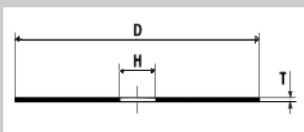
Forma BF41: egyenes
