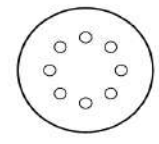
GLS 5 Ø 125 mm 8 db Ø 10 mm elszívólyuk Ø 65 mm lyukkörön
