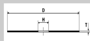
Forma BF41: egyenes
