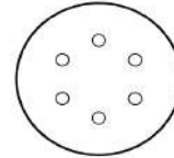
GLS 3 Ø 150 mm 6 db Ø 10 mm elszívólyuk Ø 80 mm lyukkörön
