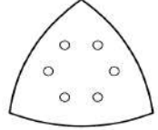
GLS 15 Ø 96 mm háromszög 6 db Ø 8 mm elszívólyuk Ø 52 mm lyukkörön
