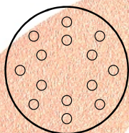
GLS 6 Ø 150 mm 8 db Ø 10 mm elszívólyuk Ø 118 mm lyukkörön 6 db Ø 10 mm elszívólyuk Ø 80 mm lyukkörön
