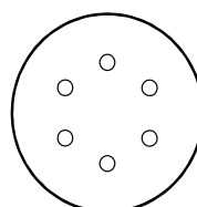
GLS 3 Ø 150 mm 6 db Ø 10 mm elszívólyuk Ø 80 mm lyukkörön
