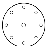
GLS 1 Ø 150 mm 8 db Ø 10 mm elszívólyuk Ø 120 mm lyukkörön + 1 db 17 mm központi lyuk
