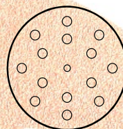
GLS 6 Ø 150 mm 8 db Ø 10 mm elszívólyuk Ø 118 mm lyukkörön 6 db Ø 10 mm elszívólyuk Ø 80 mm lyukkörön + 1 db 7 mm központi lyuk
