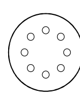
GLS 4 Ø 115 mm 8 db Ø 10 mm elszívólyuk Ø 65 mm lyukkörön
