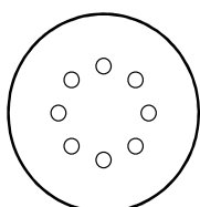
GLS 2 Ø 150 mm 8 db Ø 10 mm elszívólyuk Ø 65 mm lyukkörön
