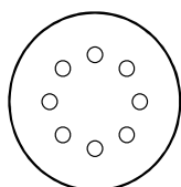
GLS 5 Ø 125 mm 8 db Ø 10 mm elszívólyuk Ø 65 mm lyukkörön
